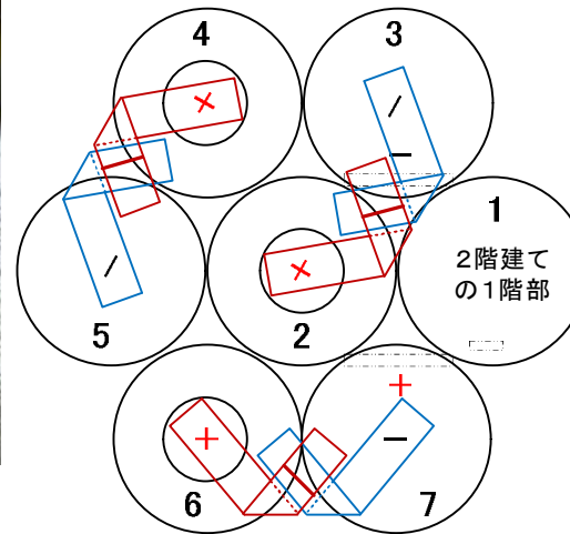
両方とも上から見たところ、平面図示略図
